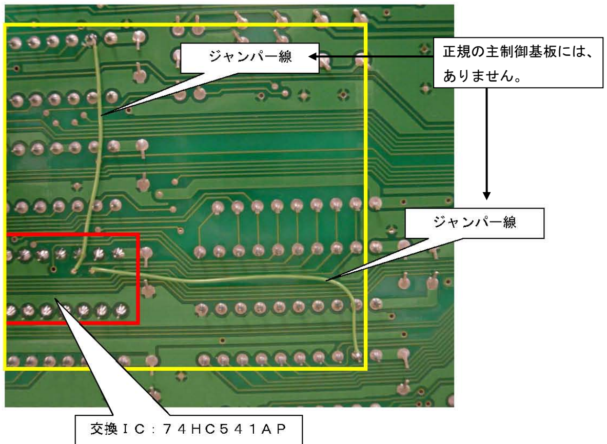
【図4】主制御基板(裏面)拡大
