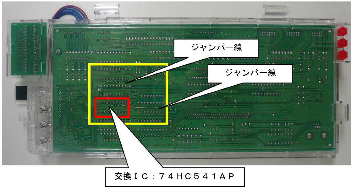
【図3】主制御基板(裏面)全体
