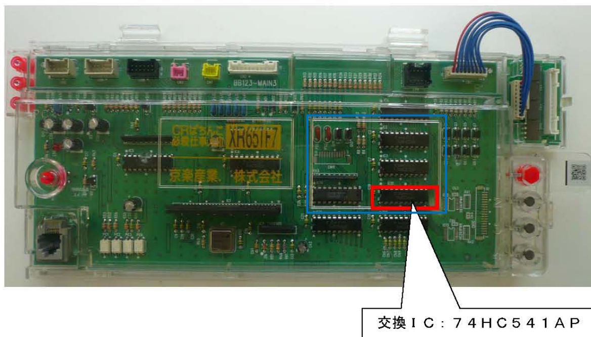
【図1】主制御基板(表面)全体
