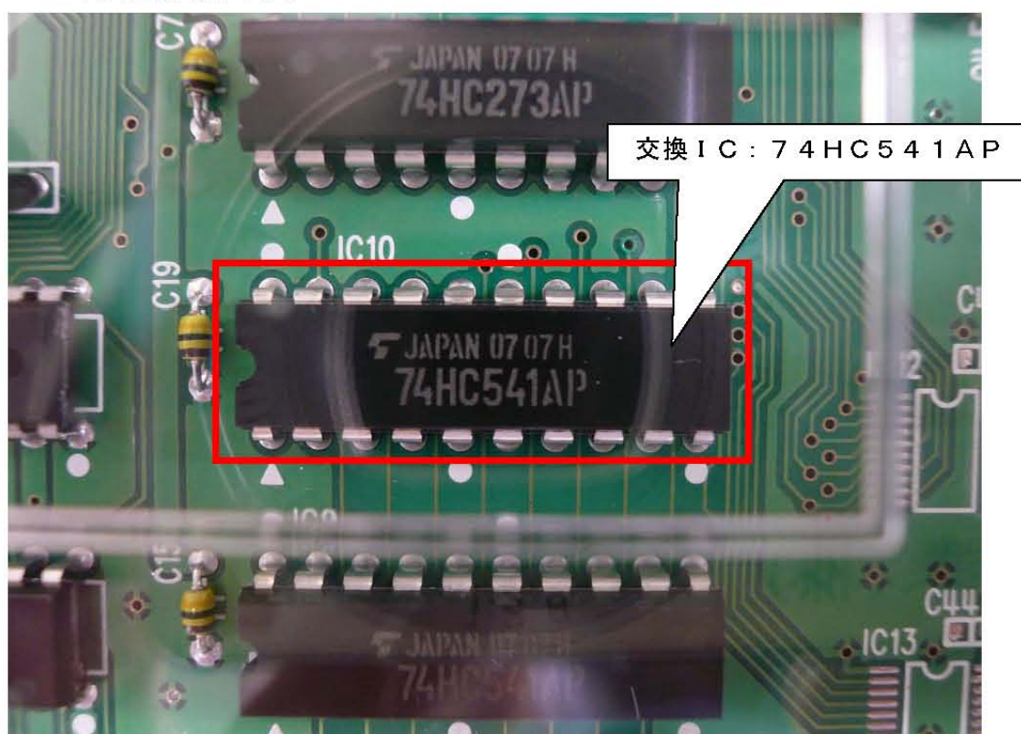
【図2】主制御基板(表面)拡大
